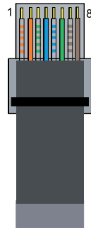
EIA/TIA 568B
