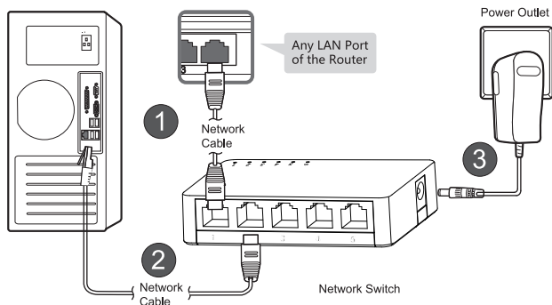
장치 연결 다이어그램
